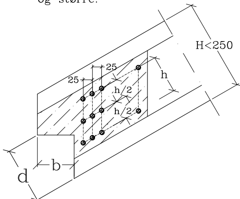
Fig 2. Tre spikerrekker for bjelke dimensjoner mindre enn 250 mm. Forøvrig samme mål som for større bjelker.
