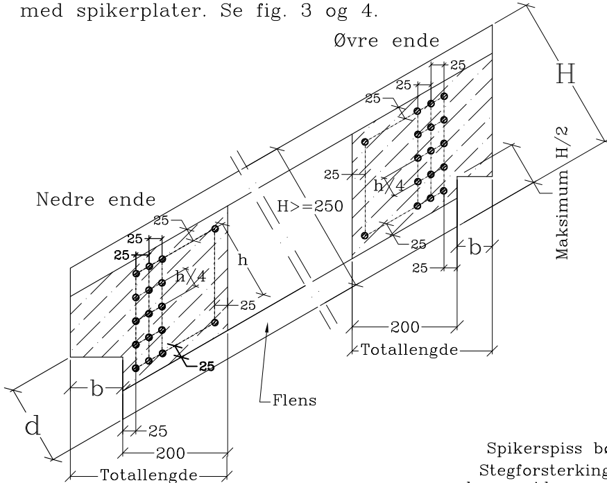
Fig 1. For garp der flens kappes helt bort av loddkutt. Bjelke dimensjon 250 mm og større.
